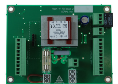
AFF/001 Flash'n'Fill™ PCB
